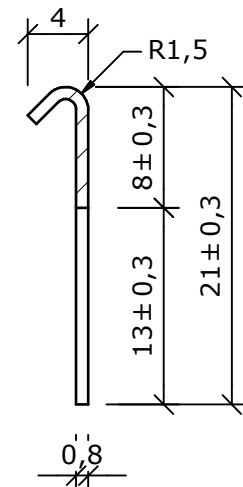
Schnitt B-B (2 : 1)
