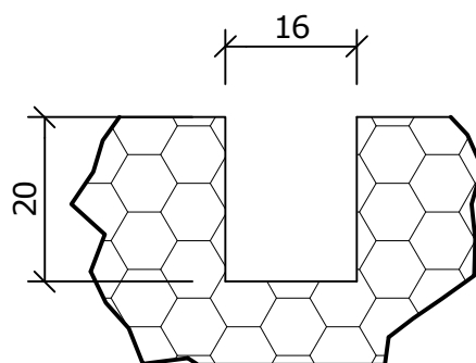
Detail X ( 1 : 1 )
