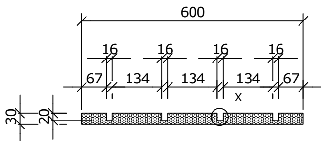
Schnitt A-A ( 1 : 10 )
