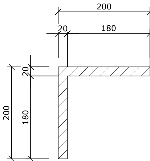
Schnitt A-A ( 1 : 5 )
