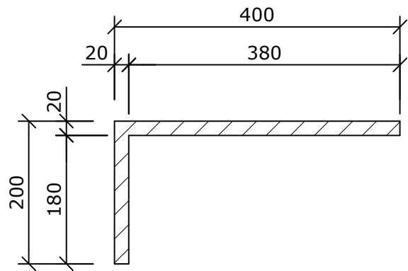
Schnitt A-A ( 1 : 7,5 )
