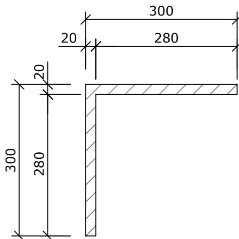
Schnitt A-A ( 1 : 7,5 )
