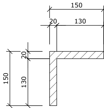
Schnitt A-A ( 1 : 5 )
