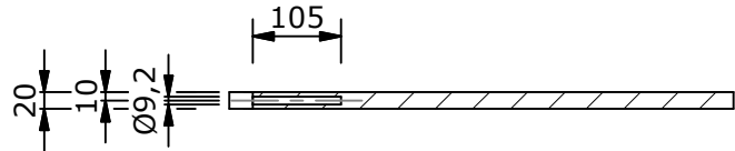
Schnitt A-A (1 : 10)
